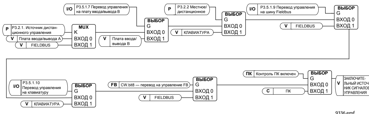
Рис. 28. источник сигналов управления
