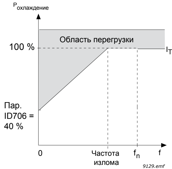
Рис. 77. Кривая теплового тока I_T двигателя, ИД 706 = Р3.9.2.3 Коэффициент ухудшения охлаждения при нулевой скорости
