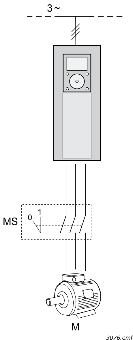
Рис. 47. Коммутатор двигателя
